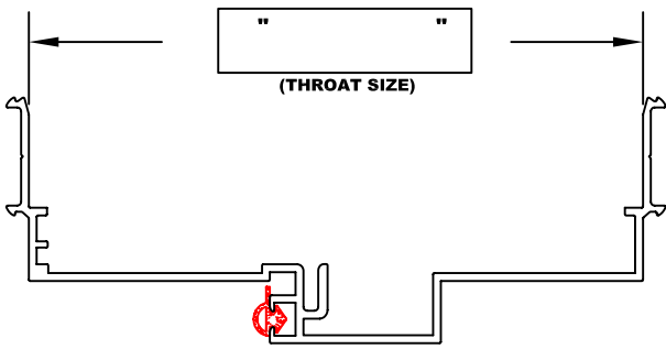
ABS-AC - STD. FRAME
